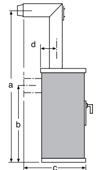
Maß a und c: mit Original-Winkelrohr dimension a and c: with original angle pipe misura a e c: con tubo ad angolo originale câtes a et c: avec conduit caudé d'origine
