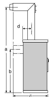
Maß a und c: mit Original-Winkelrohr dimension a and c: with original angle pipe Côtes a et c: avec conduit coudé d'origine Wymiary a i c: z oryginalną rurą pod kątem 90°
