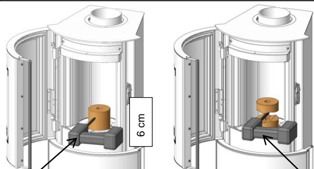
Fig. 2 et 3: préparer la briquette visseuse électrique avec outil brise-bûches
