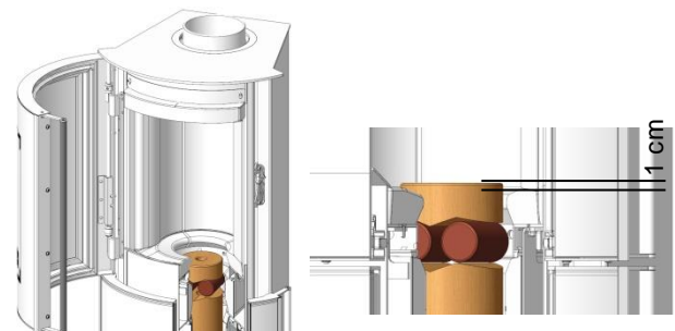
Fig. 5: Startposition: Höhe siehe Detail rechts.
